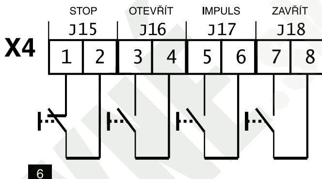
Zapojení ovládacích prvků OTEVŘÍT; STOP; ZAVŘÍT a IMPULS
