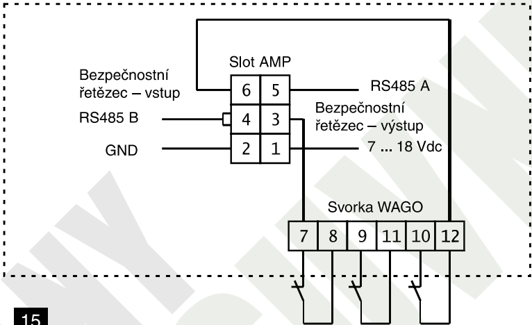
Rozložení slotů a svorek
