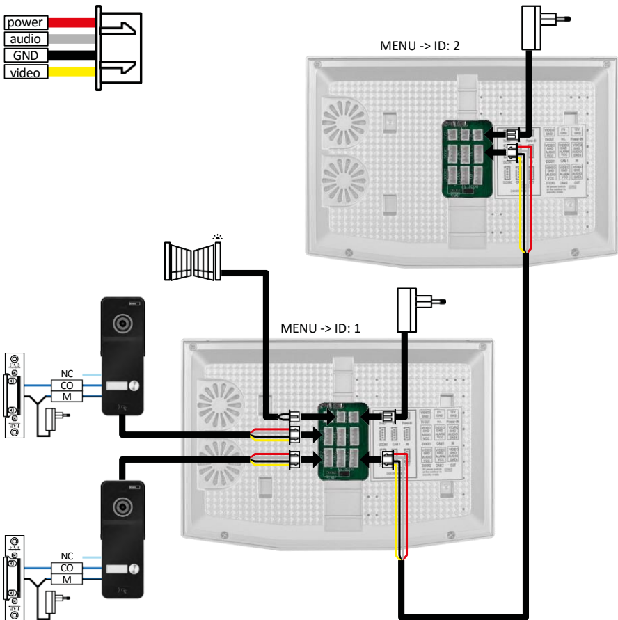
2x vonkajšie jednotky + hlavný monitor (DOOR1+DOOR2) + podriadený monitor
